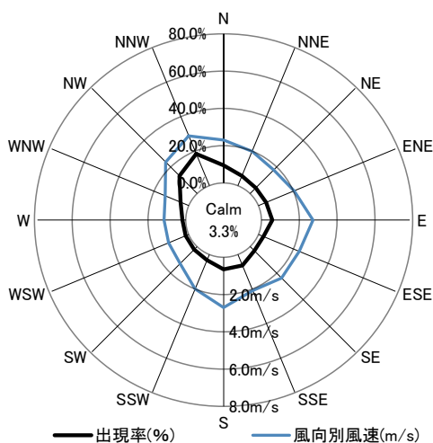
図 3.1-7 風配図 (既存調査)
