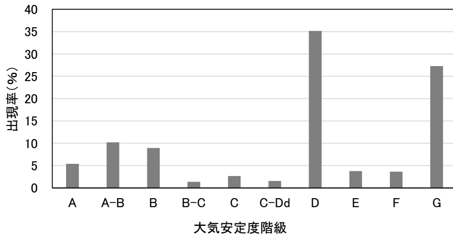
図 3.1-9 大気安定度階級の出現率
